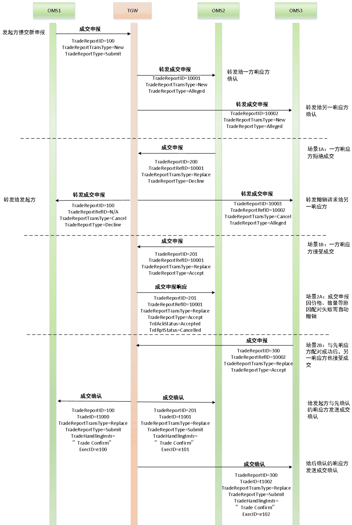
图 3-20 新成交申报处理消息流示意图
