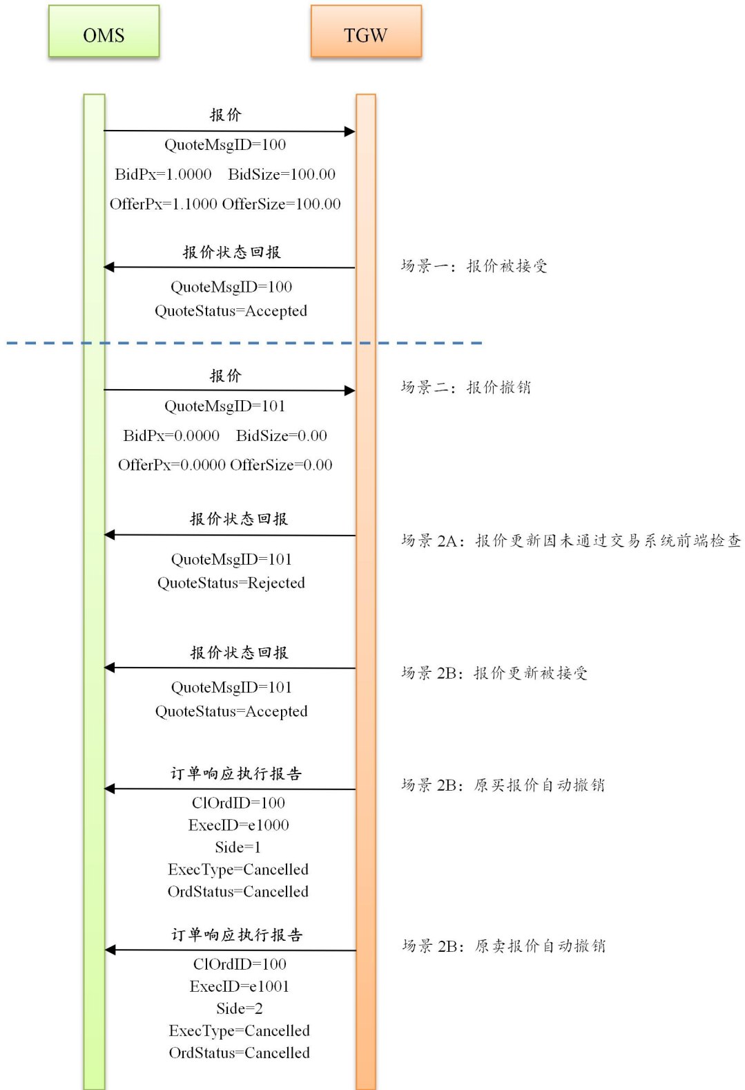
图 3-7 报价撤销处理消息流示意图
