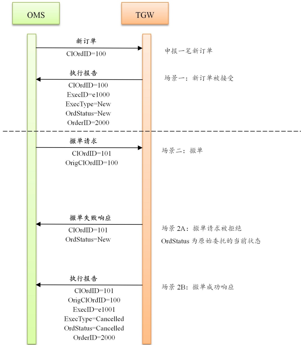
图 3-2 撤单请求消息流示意图
