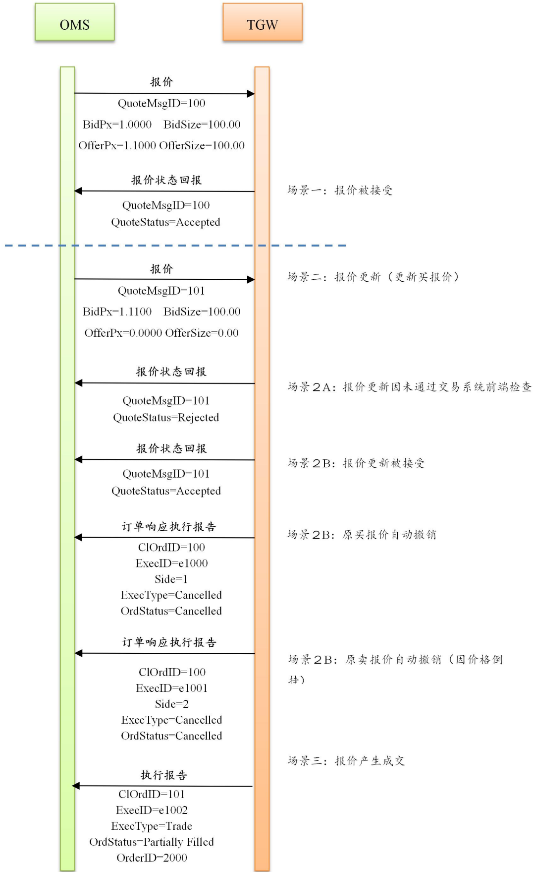
图 3-6 更新单边报价（情形三）处理消息流示意图
