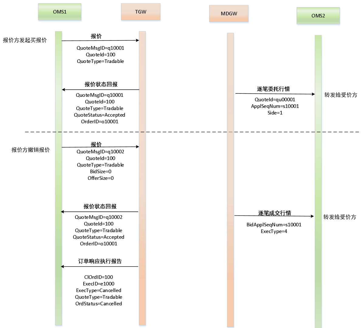
图 3-9 报价方撤销报价处理消息流示意图
