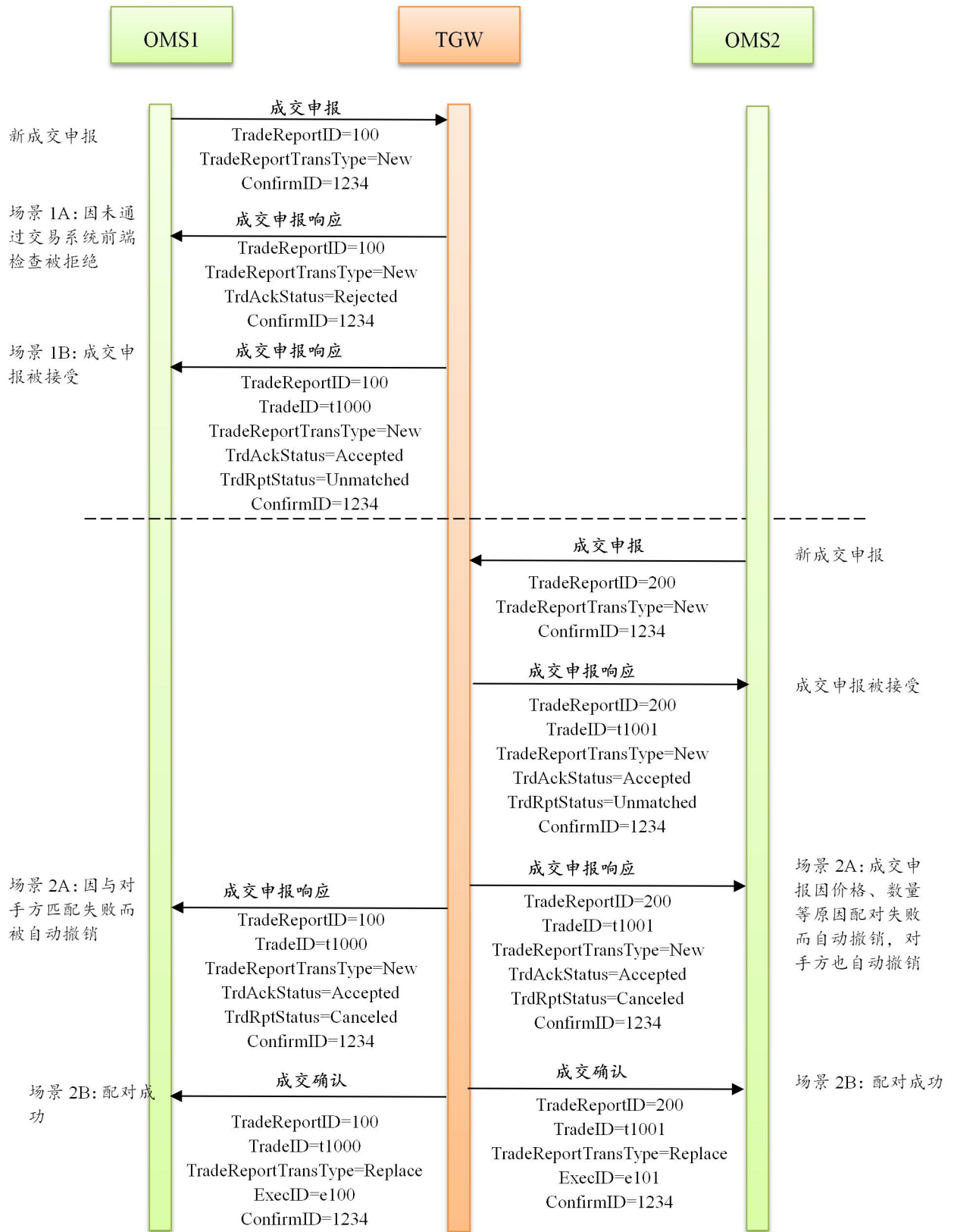
图 3-14 新成交申报处理消息流示意图
