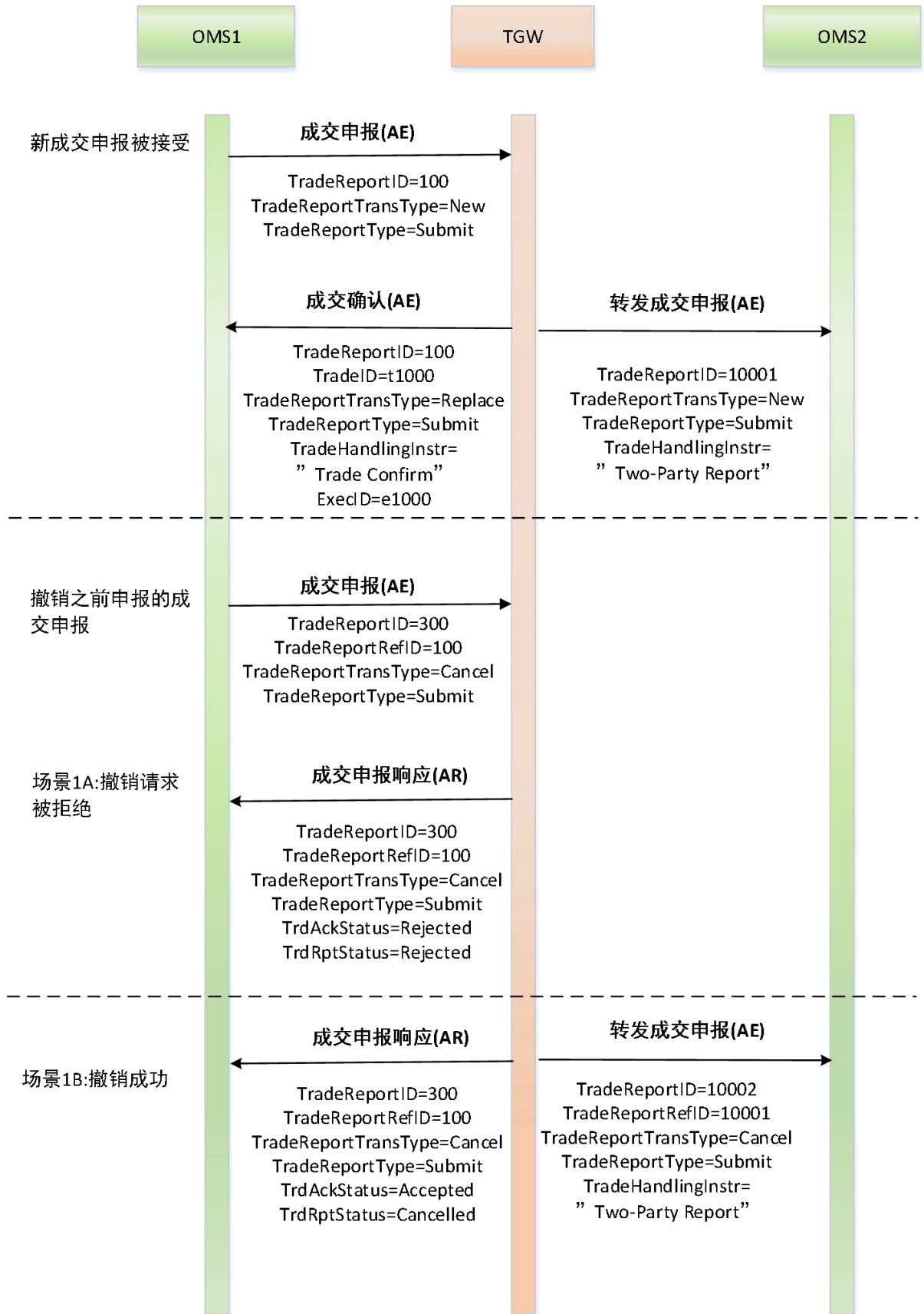
图 3- 17 成交报告撤销成交申报处理消息流示意图
