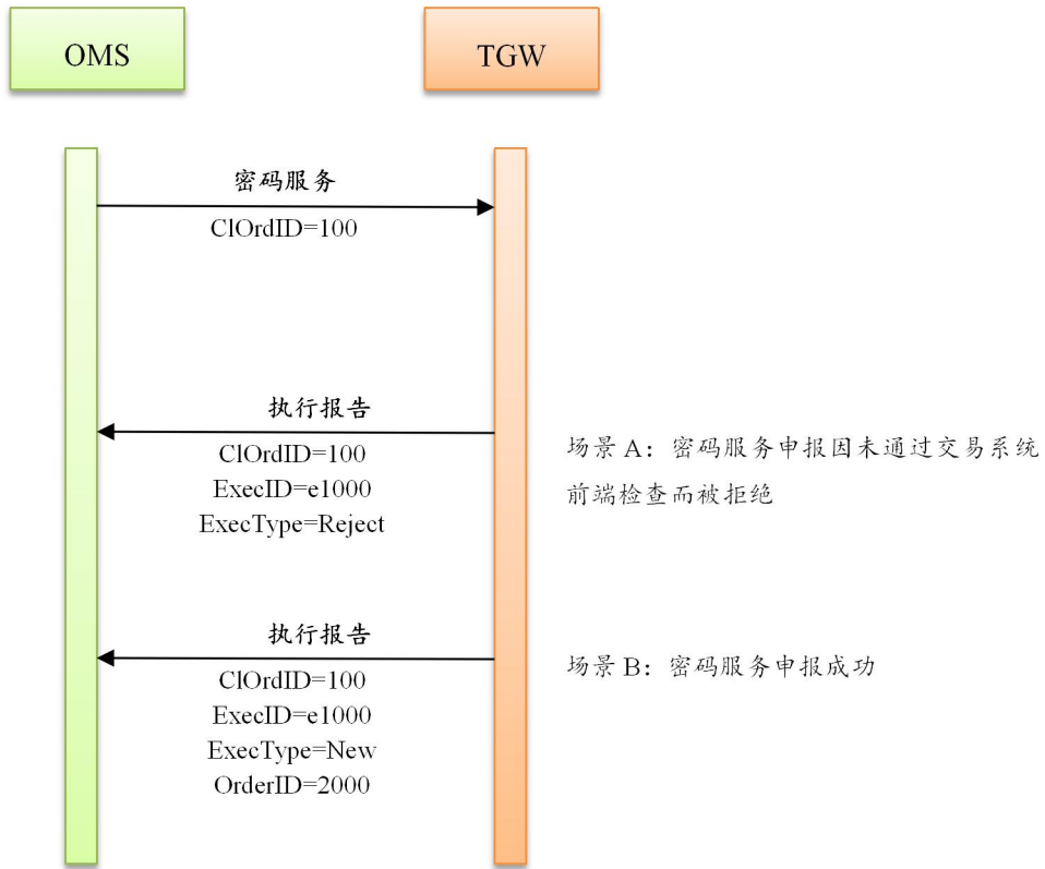
图 3-24 密码服务处理消息流示意图
