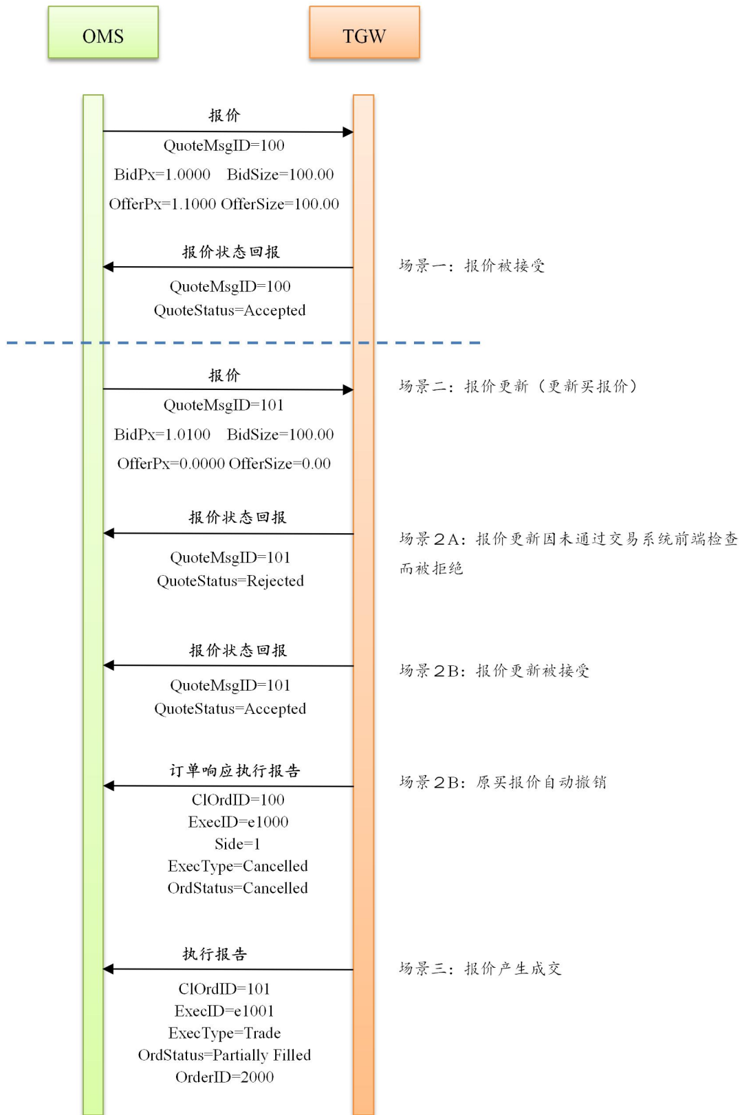
图 3-5 更新单边报价（情形二）处理消息流示意图
