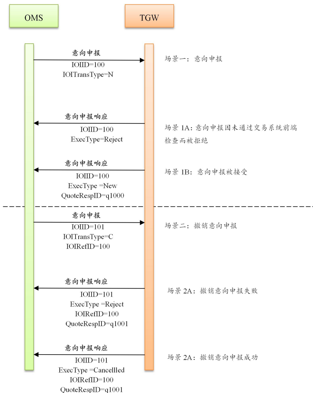
图 3-13 意向申报处理消息流示意图
